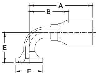
B : Cut-Off Allowance, F : Flange Dia., E : Drop Length
